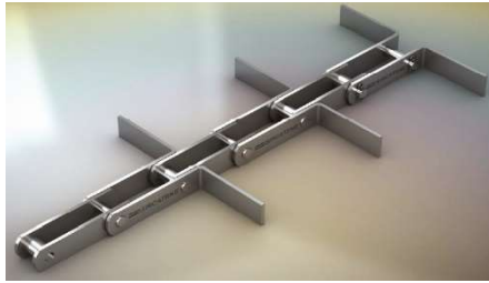
Cadena de palas según DIN 8167
